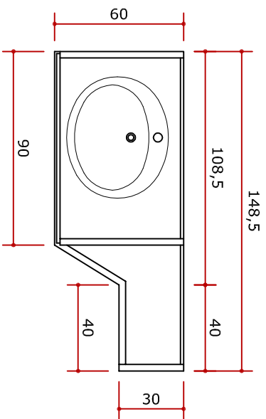
VISTA SUPERIOR
